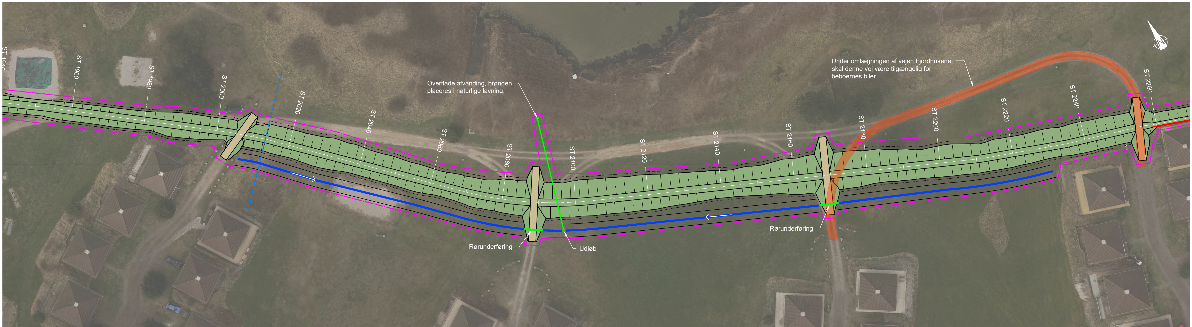
PLAN, 1:500 Fjordhusene
